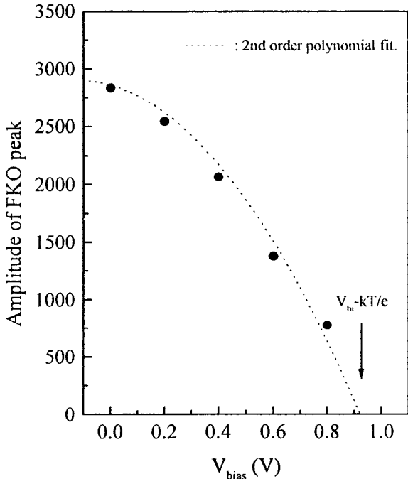
그림 7. dc 바이어스 전압( V_{bias} )와 FKO 피크 크기와와의 관계. Fig. 7. Relationship between amplitude of FKO peak and dc bias voltage( V_{bias} ).
