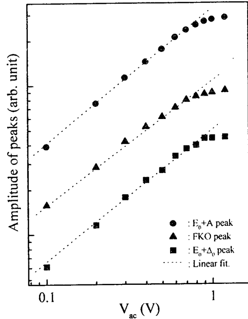
그림 2(b). Au/n-Al 0.33 Ga 0.67 As Schottky barrier diode의 ER 스펙트럼에서 변조전압에 따른 피이크의 크기.
