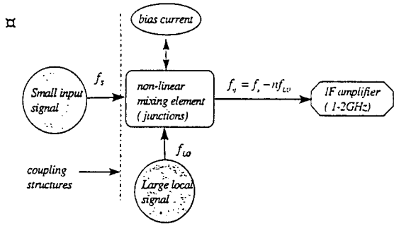
그림 29. 외부의 신호를 측정하고자 사용하는 간단한 detecting 구조 Fig. 29. Typical detecting structure for the investigation of external source
