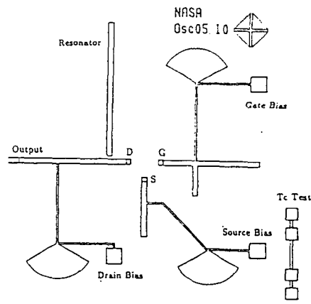
그림 20. 고온초전도 공진기와 반도체 MESFET로 구성된 oscillator Fig. 20. Hybrid oscillator made from high T c superconductors and MESFET
