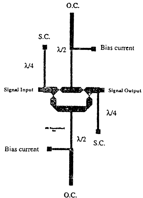
그림 16. 고온초전도체를 이용한 복합페이스 시프터 Fig. 16. Hybrid digital phase shifter using high T c superconductors
