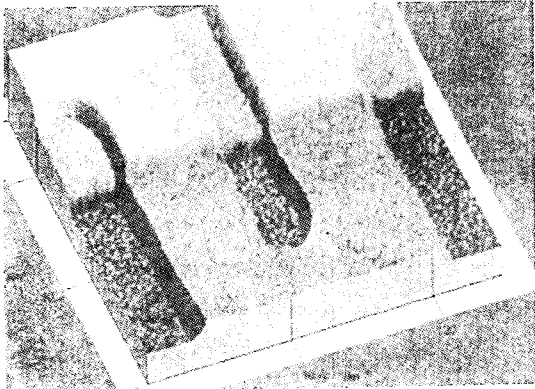
그림 25. Step-edge junction을 이용 DC-SQUID Fig. 25. DC-SQUID using step-edge junction.
