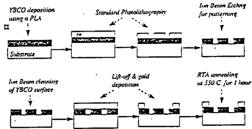
그림 6. 전형적인 고온초전도 박막 patterning process.
