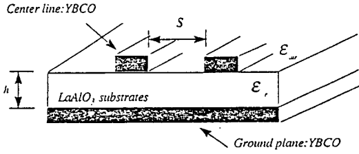
그림 9. 전형적인 고온초전도 parallel-coupled 필터의 단면
