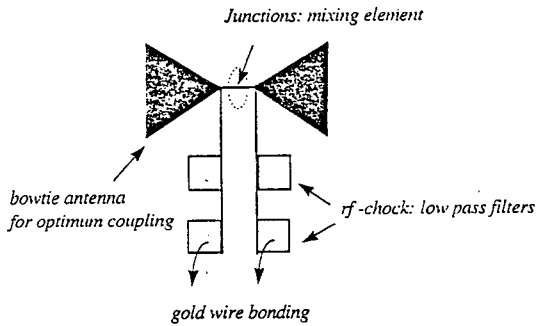
그림 30. 고온초전도 detectors Fig. 30. High T c superconducting detectors.
