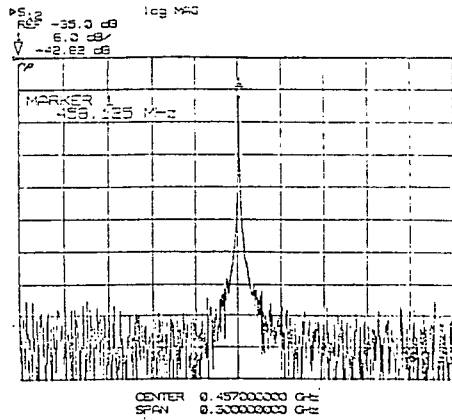
그림 7. 전형적인 공진기의 transmission data. Fig. 7. Typical transmission data of resonator.
