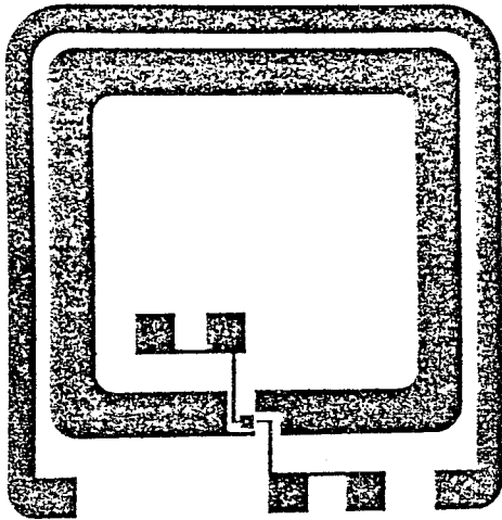
그림 27. 전형적인 Directly-coupled DC-SQUID Fig. 27. Typical Directly-coupled DC-SQUID
