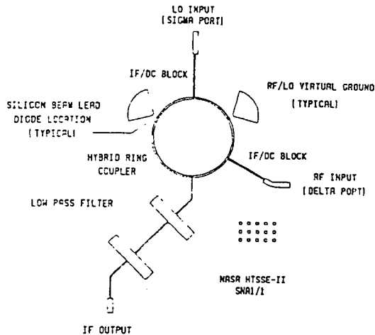
그림 31. 저주파 영역에서 사용하는 mixer Fig. 31. Low frequency mixer which is made from high T c superconducting thin films.
