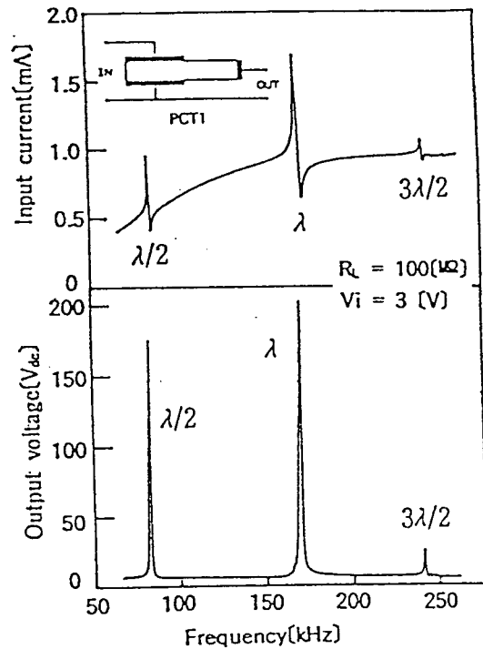
그림 4. PCT1의 공진특성
