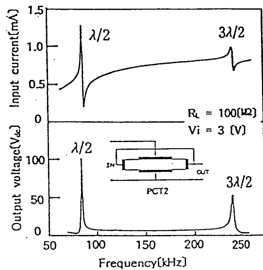
그림 5. PCT2의 공진특성
