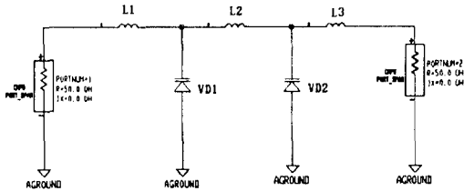
그림 10. 가변저역통과필터의 회로도 Fig. 10 Circuit schematic of tunable low-pass filter
