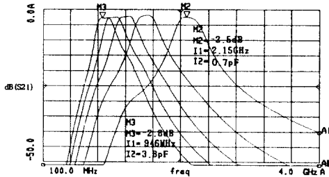
그림 18. 기생성분을 고려한 가변대역통과필터의 시뮬레이션 특성
