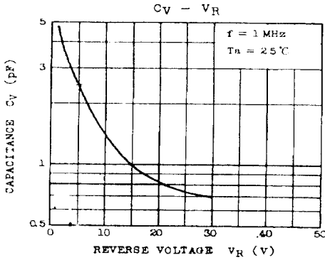
그림 2. ISV186의 C_V - V_R 특성 Fig. 2 C_V - V_R characteristics of ISV186 [8]
