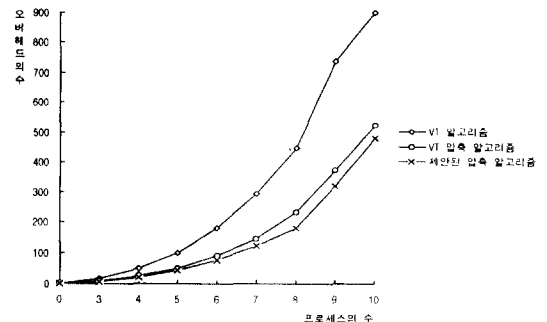
그림 5. 다른 지연 타이머를 사용할 때 메시지 오버헤드의 비교 Fig. 5 Comparison of the message overhead with the different delay timer
