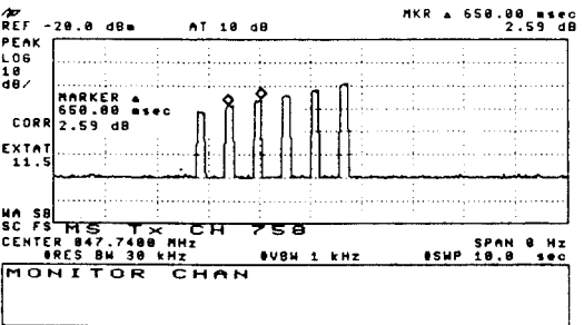
(c) PWR_STEP=5 일 때 전력 증분 측정치
