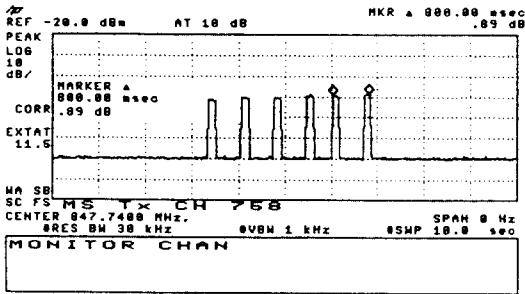
(a) PWR_STEP=1 일 때 전력 증분 측정치
