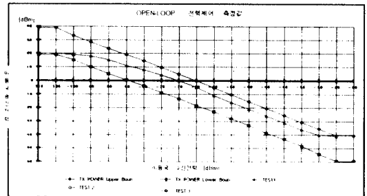
그림 5. 개루프 전력제어 측정값
