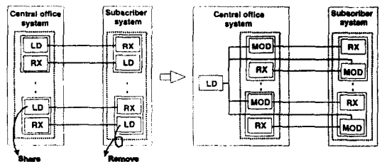
그림 1. 공유광원 및 원격변조방식을 채택한 광가입자 시스템 구조
