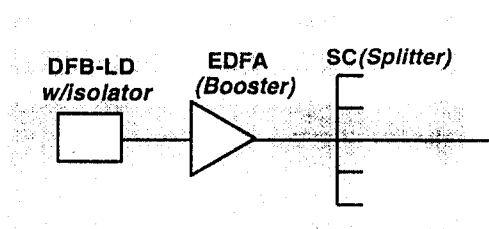
a) 공유레이저 광원
