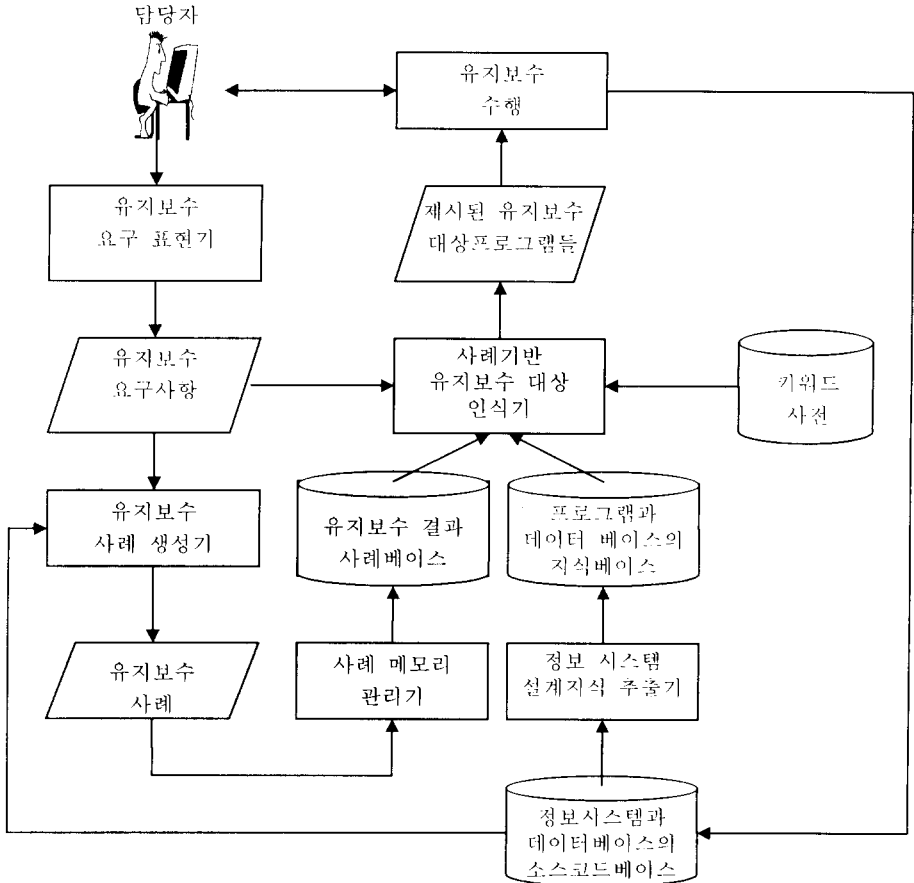
그림 1. METASOFT의 구조
