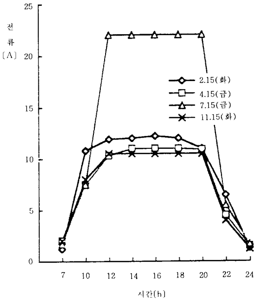
그림 1. 일 부하곡선 Fig. 1. Daily load curve
