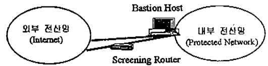
(b) 스크린 호스트 게이트웨이
