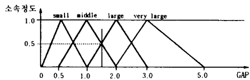
그림 5. 퍼지 집합을 이용한 각장과 갭 크기의 평가
