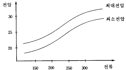
그림 2. 용접전류와 용접 전압의 상관 관계
