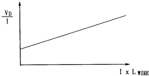
그림 3. 용접전류와 와이어 돌출길지의 상관 관계
