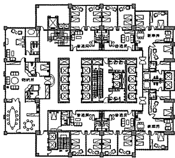
18~23층 평면도
