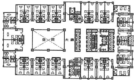
8~14층 평면도
