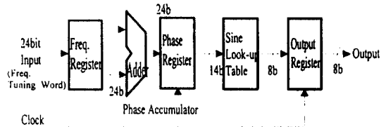
그림 1. DDFS(Direct Digital Frequency Synthesizer)의 일반적인 구조
