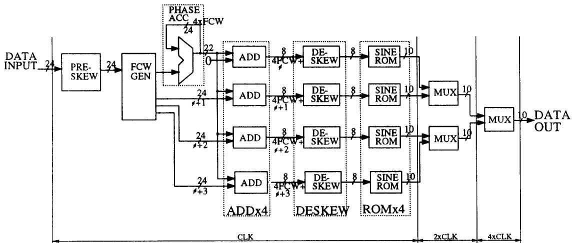
그림 2. 제안된 24-bit 병렬 구조 DDFS의 전체 블록도
