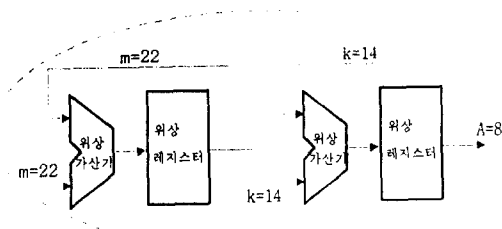
그림 5. 잡음 정형기의 블럭도 Fig. 5 Block Diagram for Noise Shaper
