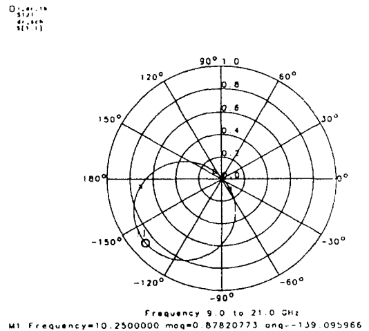
그림 3.1 유전체 공진회로 설계결과 특성 \Gamma_R Fig. 3.1 \Gamma_R of designed DR circuit
