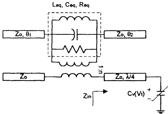
그림 2.3 유전체 공진기와 바랙터의 동가 결합구조 모델 Fig. 2.3 Equivalent coupling structure model of DR-varactor
