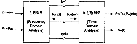
그림 2.4 HB 방법을 위한 회로 해석구조 Fig. 2.4 Analysis structure of circuit for HB method
