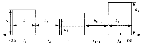
그림 1. 비대칭적인 반송파그룹의 주파수배치 Fig. 1. Unsymmetrical frequency plan of carrier groups
