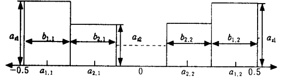
그림 2. 대칭적인 반송파그룹의 주파수배치 Fig. 2. Symmetrical frequency plan of carrier groups
