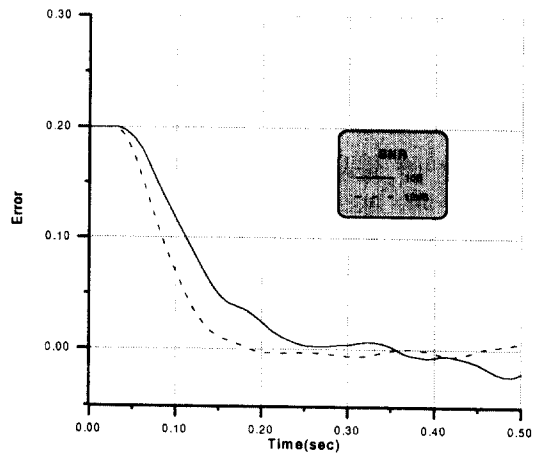
그림 8. SNR에 따른 정지 표적의 추적 성능 Fig. 8 Tracking performance of a stationary target with different SNRs.
