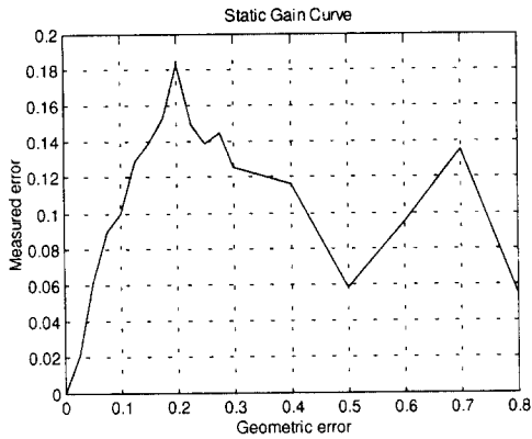
그림 4. 고정 레티클 탐색기의 정적이득특성 Fig. 4 Static gain curve of the fixed reticle seeker.
