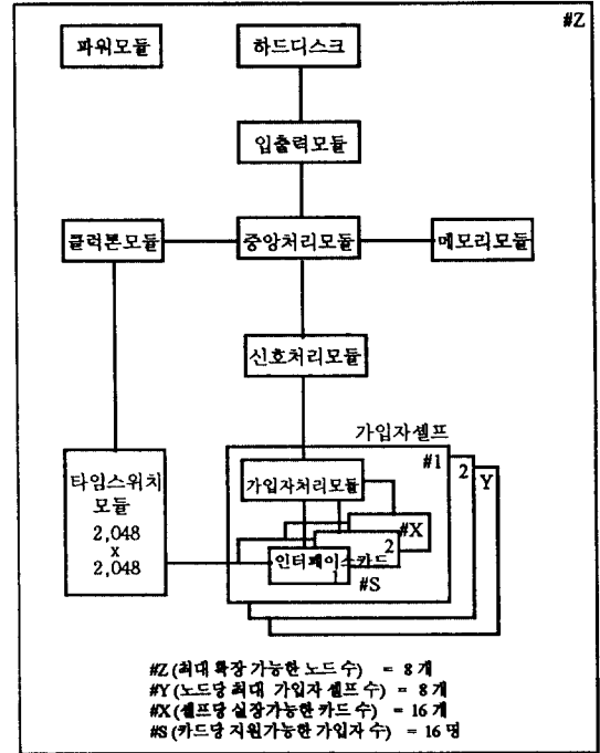
그림 1. ISDN 사설교환기의 전체 구조 Fig. 1 Whole structure of the ISDN PABX
