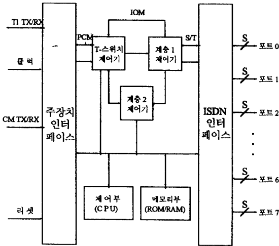
그림 2. ISDN 카드의 하드웨어 구조 Fig. 2 Hardware structure of ISDN card
