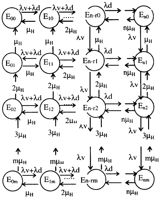
그림 4. 상태 천이도
