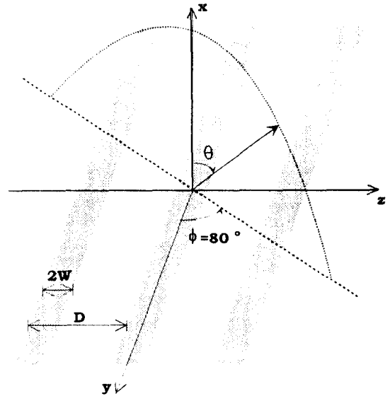
그림 5. 누설파의 진행방향과 산란특성을 기술하기 위한 좌표계
