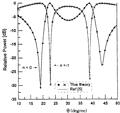
그림 4. \theta 에 대한 산란파상대전력 P_{n=0} , P_{n=-1} ( \epsilon_r = 2.57 , D = \lambda , 2W = 0.188D , h/D = 0.511219 , \phi = -80^\circ , \gamma = 11.5655^\circ )
