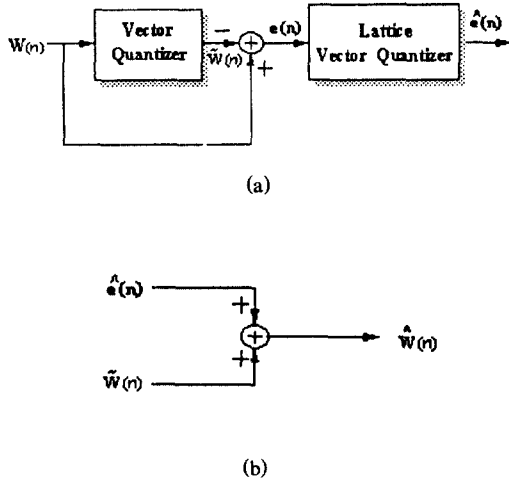
그림 3. 2단 벡터양자화의 블럭도 (a) 부호기 (b) 복호기 Fig. 3 Block diagram of two-stage vector quantizer (a) encoder (b) decoder
