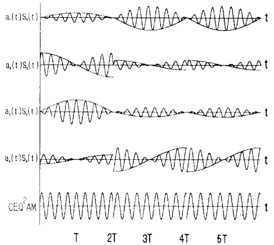
그림 7. a_i(t) 와 결합된 정진폭(Constant Envelope: CE) Q^2AM 의 데이터 성형 펄스 및 파형
