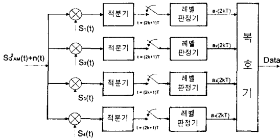
그림 3. Q 2 AM 복조 시스템
