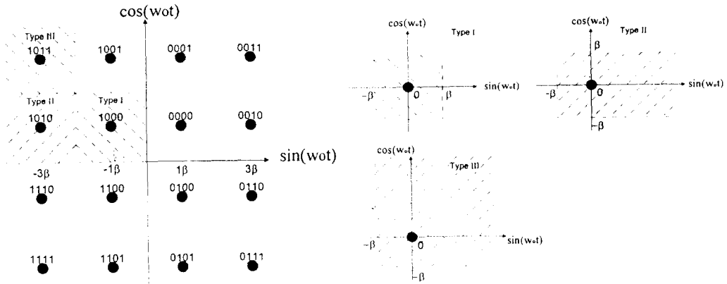
그림 4. 기저대역상에서의 Q²AM 신호 공간도 및 Type I~III
