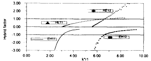
그림 3-2. 모드별 하이브리드 요인 Fig. 3-2 Hybrid mode factor
