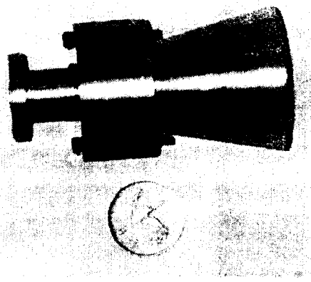
그림 9. 제작된 Ka 대역 코리게이트 혼 안테나 사진 Fig. 9 Photograph of fabricated corrugated horn antenna for Ka band
