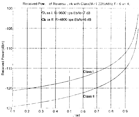
그림 1. 기지국에서의 전력변화 Fig. 1 The received power at the base station
