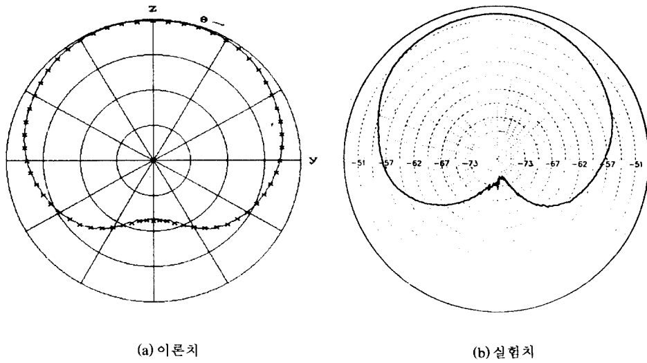
그림 11 대칭 기생소자를 갖는 마이크로스트립 안테나의 복사 패턴
