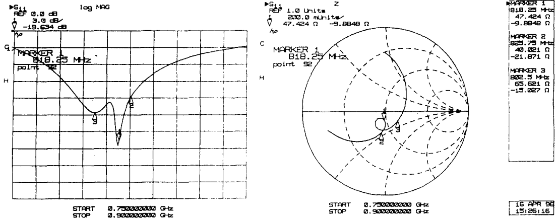
그림 9 비대칭 기생소자를 갖는 마이크로스트립 안테나의 반사손실과 입력 임피던스(실험치)
