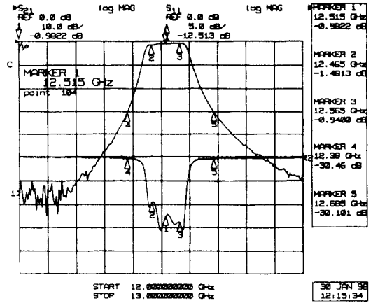
그림 14. 듀플렉서의 TX 특성
