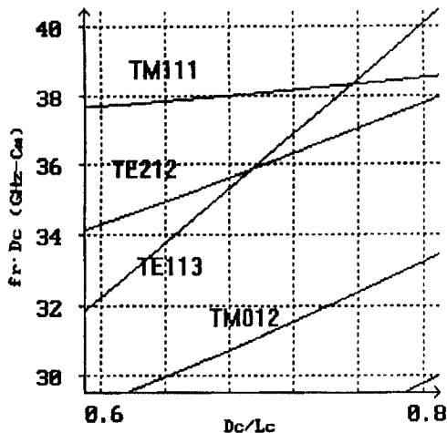
그림 6. 원통형 공동 공진기의 모드 chart Fig. 6. Mode-chart for cylindrical cavity resonator
