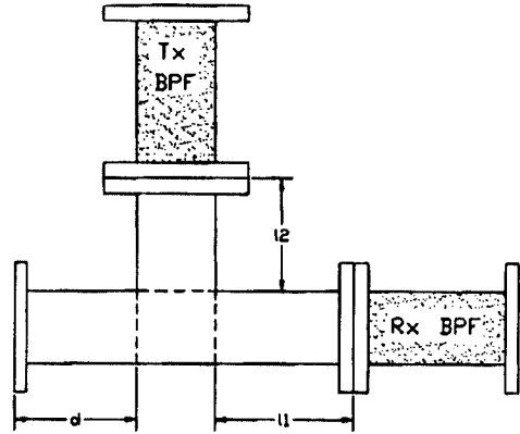
그림 4. 듀플렉서의 구성 Fig. 4. Design of the duplexer
