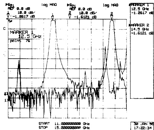
그림 13. 듀플렉서의 전체적인 응답
