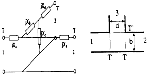
그림 5. H-면 T-접합의 등가회로 Fig. 5. Equivalent circuit of H-plane T-junction
