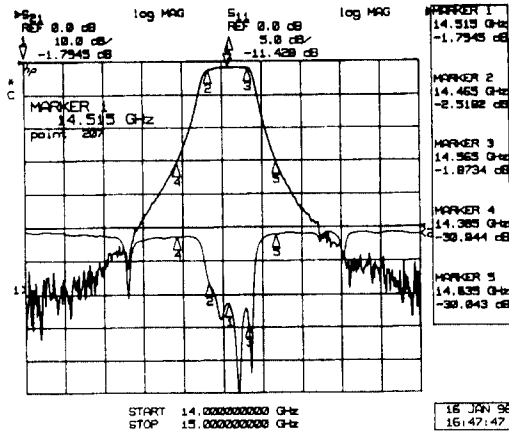
그림 12. H-면 T-접합 연결 후 14.5GHz 필터 응답 (No tuning)
