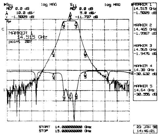
그림 15. 듀플렉서의 RX 특성
