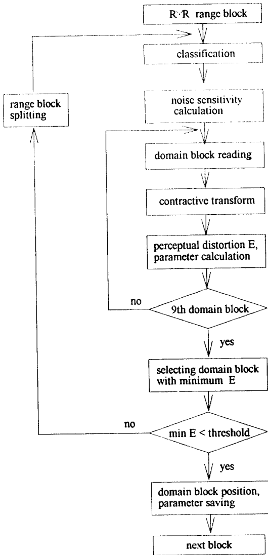
그림 4. 하나의 지역 블록에 대한 제안 알고리즘의 순서도 Fig. 4 The flow chart of the proposed algorithm for a range block
