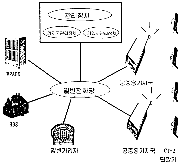
그림 1. CT-2 망구성도
