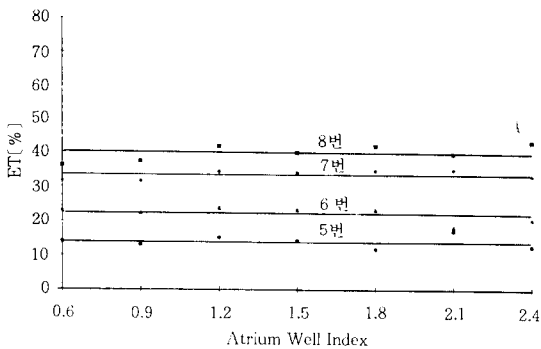
그림 13. 청천공상태에서 4-Unit 툽날형창호의 유효투과율
