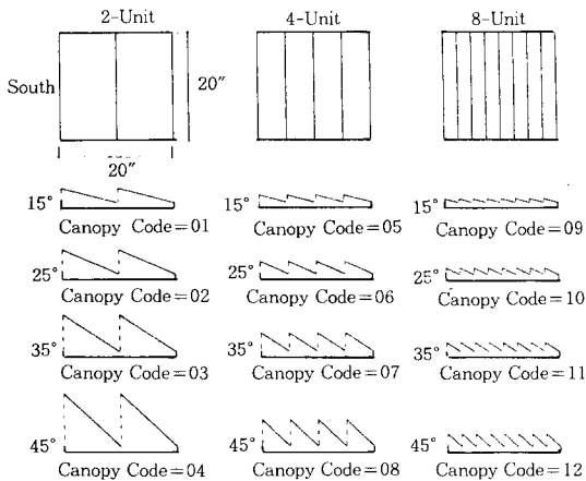
그림 9. 틈날형 아트리움 창호의 제원
