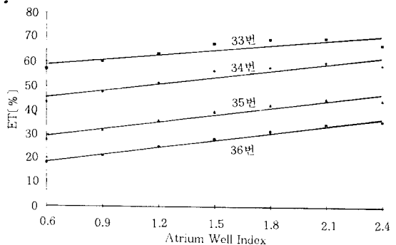
그림 16. 담천공상태에서 85% 표면반사율의 다중광정형 창호의 유효투과율
