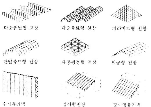
그림 4. 아트리움 창호방식의 분류
