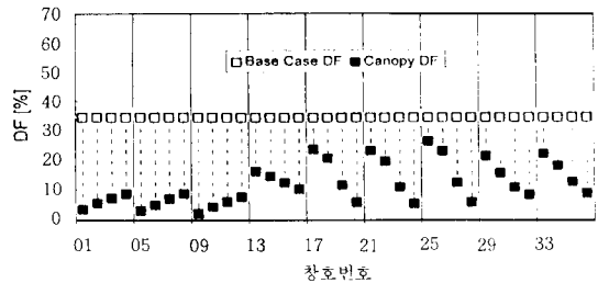
그림 12. 개방된 4면형 아트리움의 BCDF와 창호를 설치한 DF(아트리움 WI=1.2일 경우)
