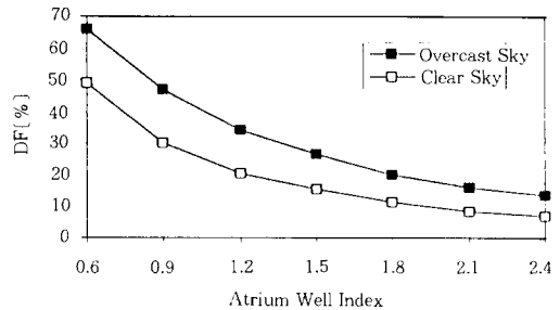
그림 11. 창호가 설치되지 않은 4면형 아트리움 바닥 중앙점에서의 주광률(BCDF)
