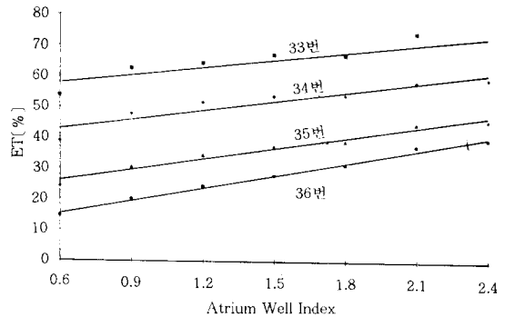
그림 15. 청천공상태에서 85% 표면반사율의 다중광정형 창호의 유효투과율
