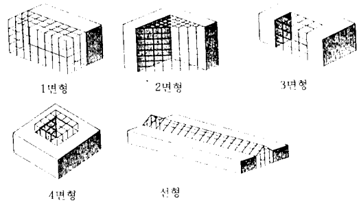
그림 3. 아트리움 방식의 분류
