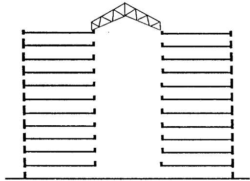
그림 1. 전형적인 아트리움 건물의 단면
