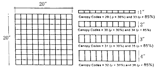
그림 10. 다중광정형 아트리움 창호의 제원
