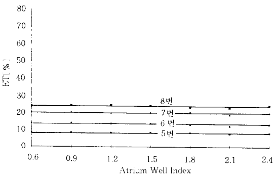
그림 14. 담천공상태에서 4-Unit 툽날형창호의 유효투과율
