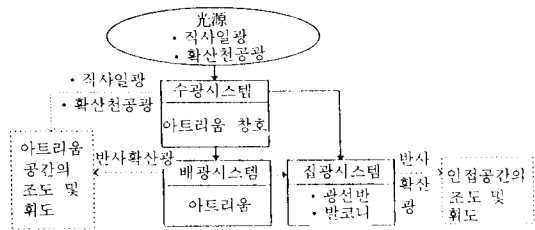
그림 2. 아트리움 건물의 자연채광 시스템들의 상호관계
