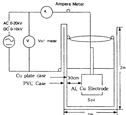
그림 5. 전기적 특성 실험 회로 및 장치
