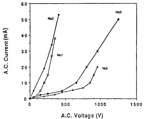
그림 10. 교류 전압 증가에 따른 교류 전류의 변화
