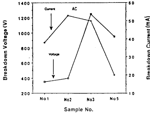
그림 11. 교류 블레이크다운 전압 전류 변화 Fig. 11. Variation between AC breakdown voltage and current
