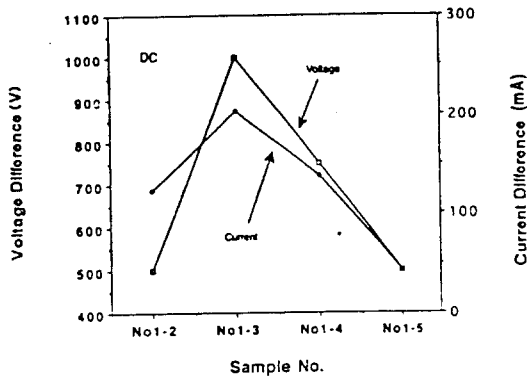
그림 8. 알루미늄 전극을 기준으로 한 직류 전압 전류 비교
