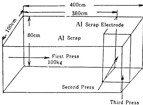
그림 4. 유압기 내부 구조
