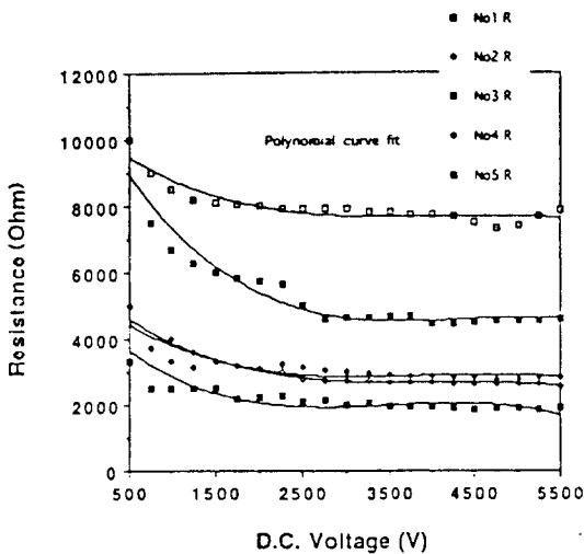
그림 9. 직류 전압 증가에 따른 접지 저항의 변화
