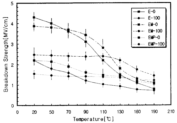
그림 5. 망목 구조 변화에 따른 시편의 교류 절연파괴강도(충진제 함량 0, 100[phr]) Fig. 5. AC dielectric strength due to variation of network structure(filler content 0, 100[phr])
