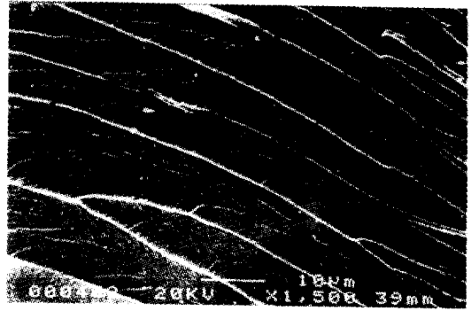
사진 2. EM-0 시편의 전자 현미경 사진 Photo. 2. SEM of EM-0 specimen.
