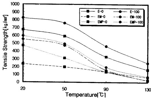
그림 6. 망목 구조 변화에 따른 시편의 인장 강도(충진제 함량 0[phr], 100[phr])
