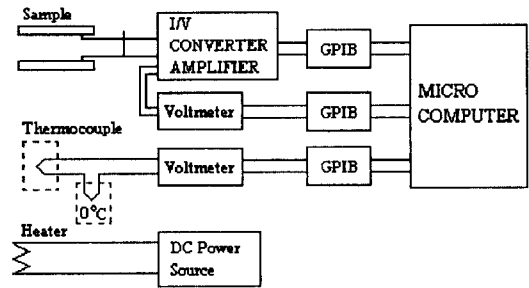
그림 3. 측정시스템 개략도
