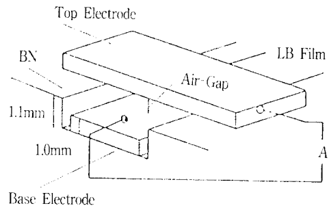
그림 4. 전극 구조
