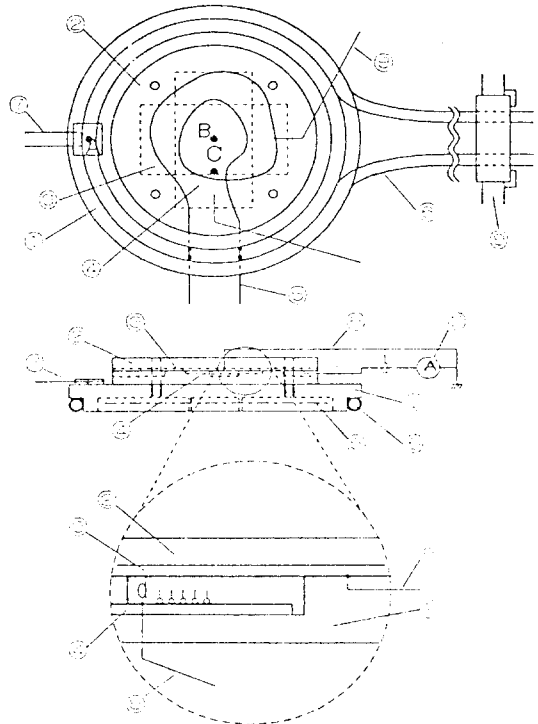
그림 2. 열자격 시스템의 구조 ① 스테인레스 판 ② BN블럭 ③ 전극 1 ④ 전극2 ⑤ 히터 ⑥ 스테인레스 튜브 ⑦ 열전 센서 ⑧ 금선 ⑨ 진공 용기 ⑩ 전류계 Fig. 2. A schematic diagram of the thermally stimulated system ① Stainless plate ② BN blocks ③ Electrode 1 ④ Electrode 2 ⑤ Heater ⑥ Stainless tube ⑦ Thermocouple ⑧ Gold wire ⑨ Vacuum vessel ⑩ Ammeter
