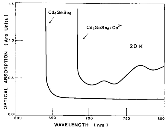
그림 1. Cd 4 GeSe 6 및 Cd 4 GeSe 6 :Co 2+ 단결정의 광흡수 스펙트라(20K)
