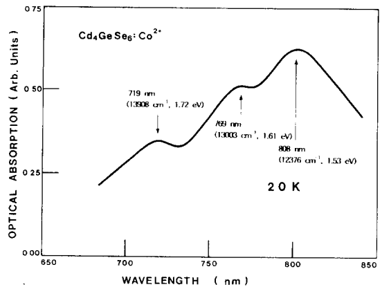
그림 3. Cd 4 GeSe 6 :Co 2+ 단결정에서 650-850nm 파장영역의 광흡수 스펙트라(20K).
