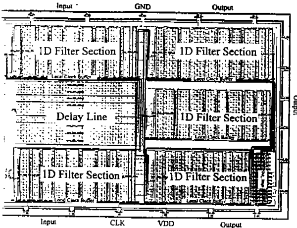
(그림 7) 2D DF 레이아웃 (Fig. 7) 2D DF layout
