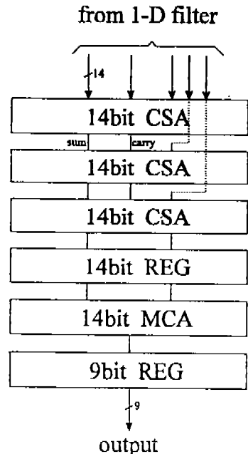
(그림 4) 출력단 (Fig. 4) Output stage
