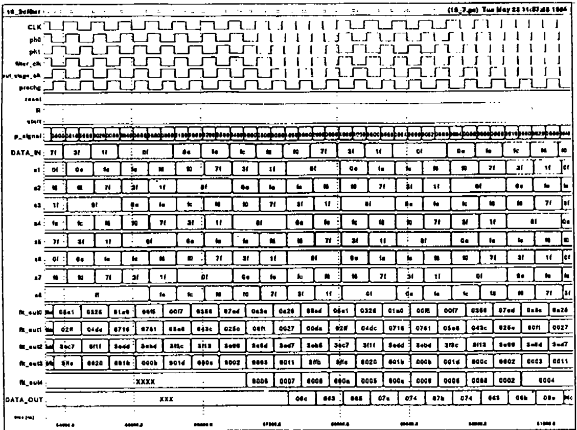
(그림 9) IRSIM 모의실험 결과의 예 (Fig. 9) Example of IRSIM simulation result
