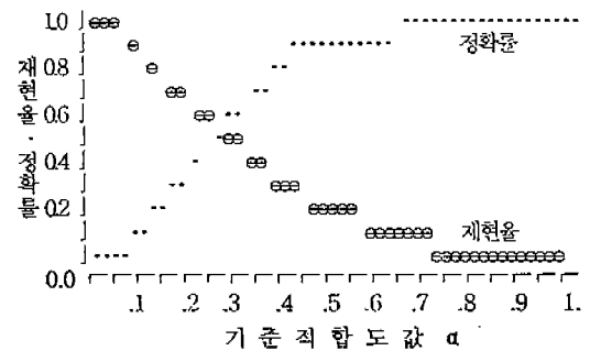
(그림 1) 색인어20과 11에서 기준적합도값, 재현율, 정확률의 관계( t_{20} \wedge t_{11} )
