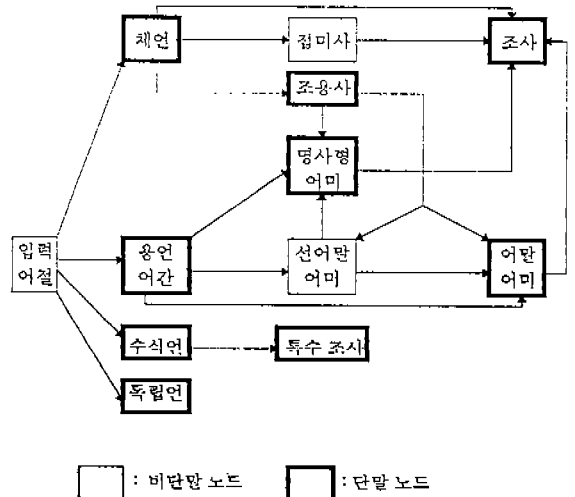
(그림 3) 한글 어절의 상태 전이도 (Fig. 3) A state diagram of Hangul Eojeol
