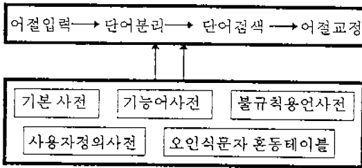
(그림 4) 전체 시스템 구성도 (Fig. 4) An overall system
