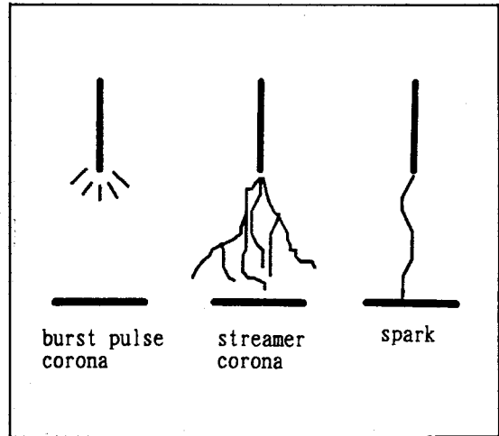
그림 3. 양극 코로나의 종류
