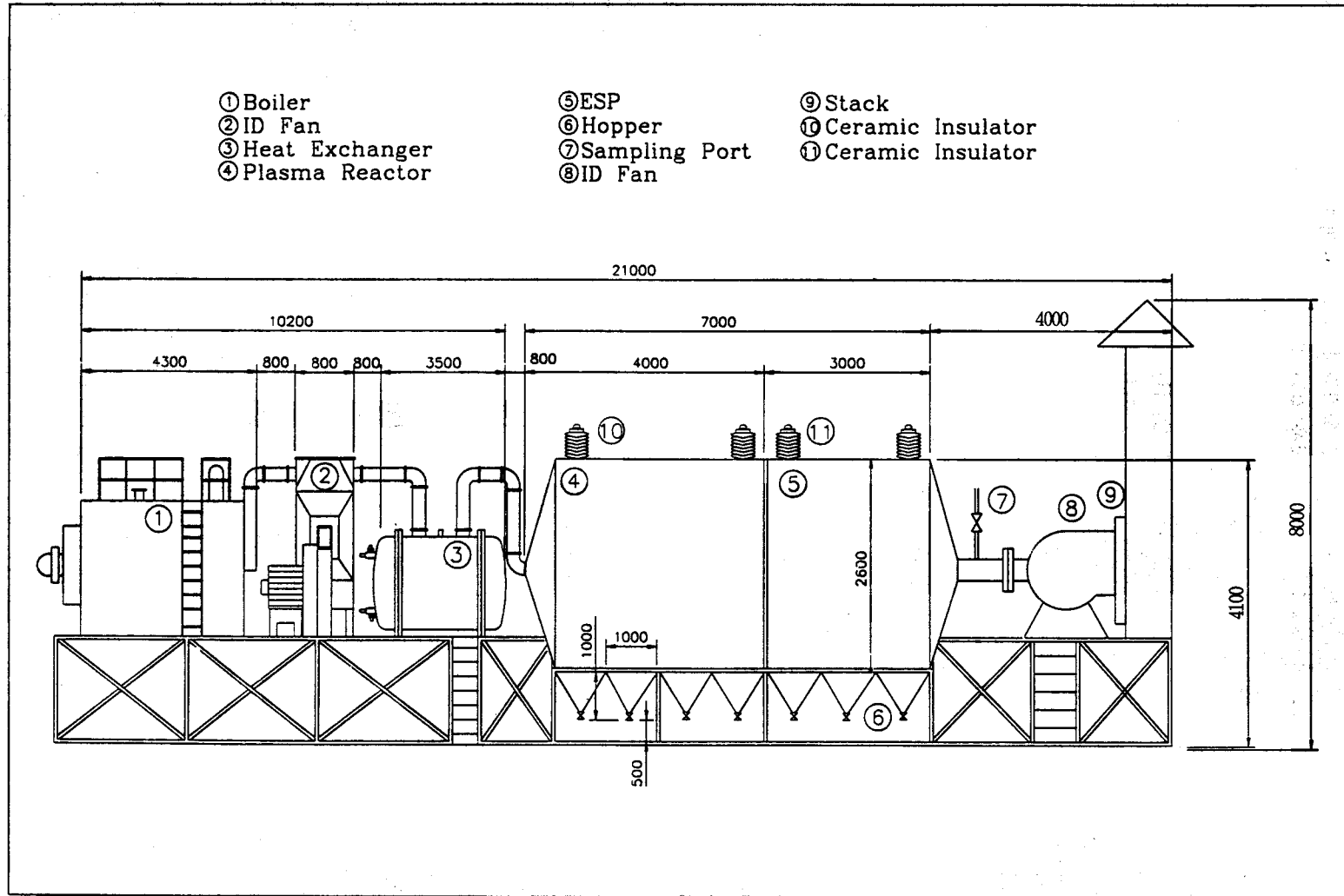
그림 5. 0.5 MW DeSOx/DeNOx SYSTEM With Plasma Reactor
