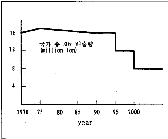
그림 2. 미국 공기청정법안에 따른 아황산가스 국가 총배출량 년도별 추이
