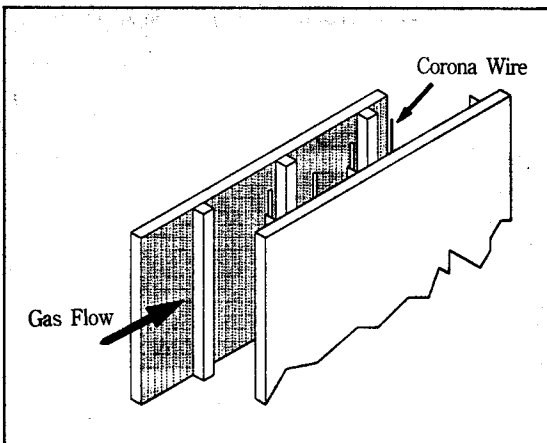
그림 7. Wire-Plate형 반응기
