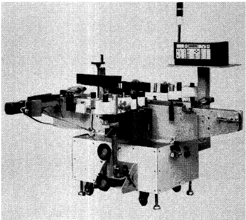
▲ 한신라벨부착기(HS6000pro)
