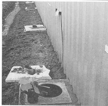
분만사 밖에 설치된 팬이 돈방 슬랫 밑으로 공기를 빼내는 음압식 공기를 채택하여 환기를 하였다.
