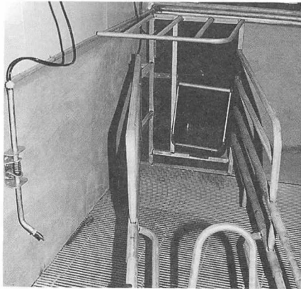
분만사 안에서 자돈들이 60일령까지 육성될 수 있도록 니플의 높이를 조절할 수 있다.
