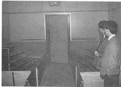
스모그 파우더를 사용하여 밖의 공기가 작은 틈을 통해 빠르게 돈사안으로 들어오는 환기 상황을 관찰하는 모습
