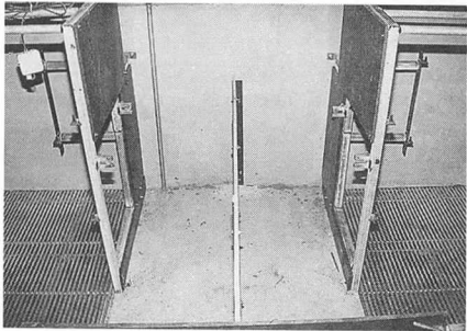
분만틀 사이에는 온돌로 되어 있어 자돈들에게 적절한 온도를 맞춰줄 수 있다.
