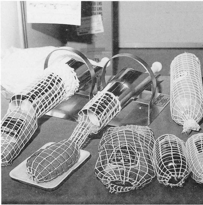
망을 이용해 육가공품 및 고기를 포장하는 기계
