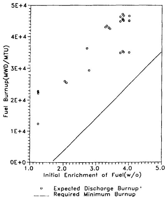
그림 1. 75% 저장밀도인 영역 2에 저장 가능한 핵연료의 최소연소도와 사용후 핵연료의 예상 방출연소도
