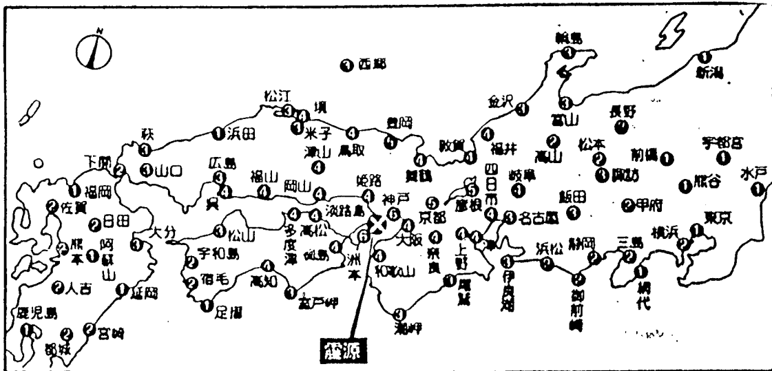
그림 1. 兵庫縣南部地震震度分布
