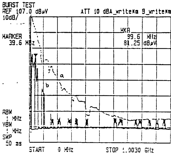
a) Level 4/500KHz에서 관통형 콘덴서만을 삽입시 감쇠특성
