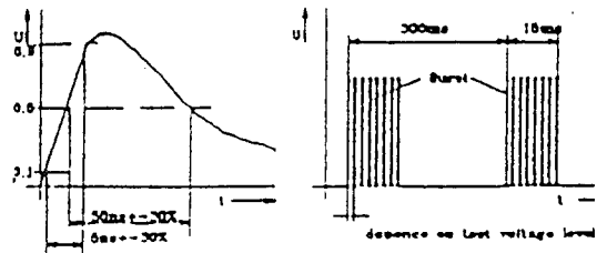
그림 1. EFT 파형정의
