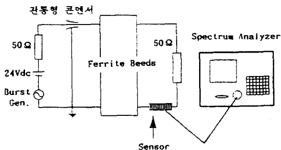
그림 3. 측정회로의 구성
