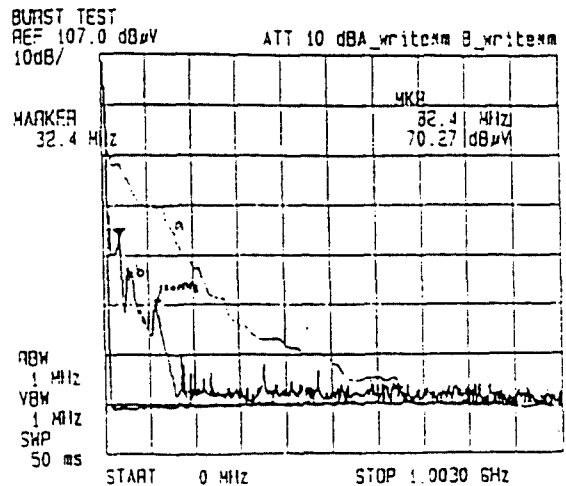
b) 관통형 콘덴서+페라이트 비드 삽입시 감쇠특성
