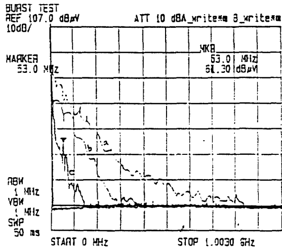
a) 관통형 콘덴서 삽입시 표준신호에서 감쇠특성
