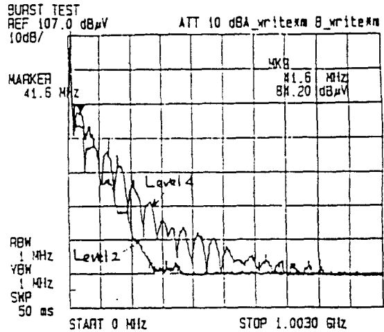
a) IEC가 정의한 Level4/2의 스펙트럼 비교(2.5KHz)
