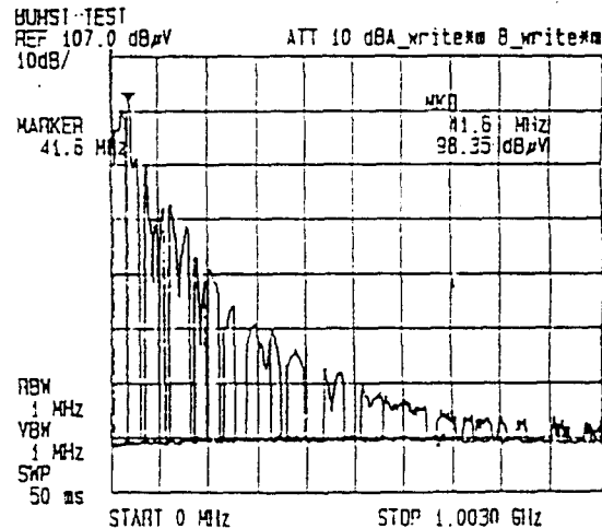
b) Level 4의 500KHz시 스펙트럼
