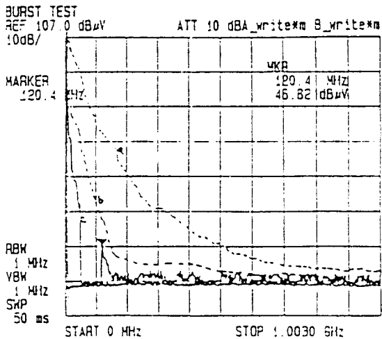
b) Level 4/500KHz에서 관통형 콘덴서 + 페라이트 비드삽입시 감쇠특성
