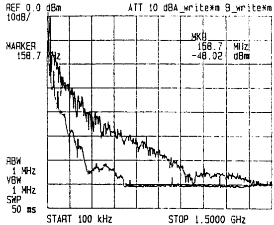
그림 8. Permalloy를 삽입시 감쇠특성
