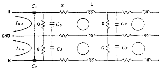
그림 5. EFT에 내성을 갖는 새로운 전원코드의 등가회로.
