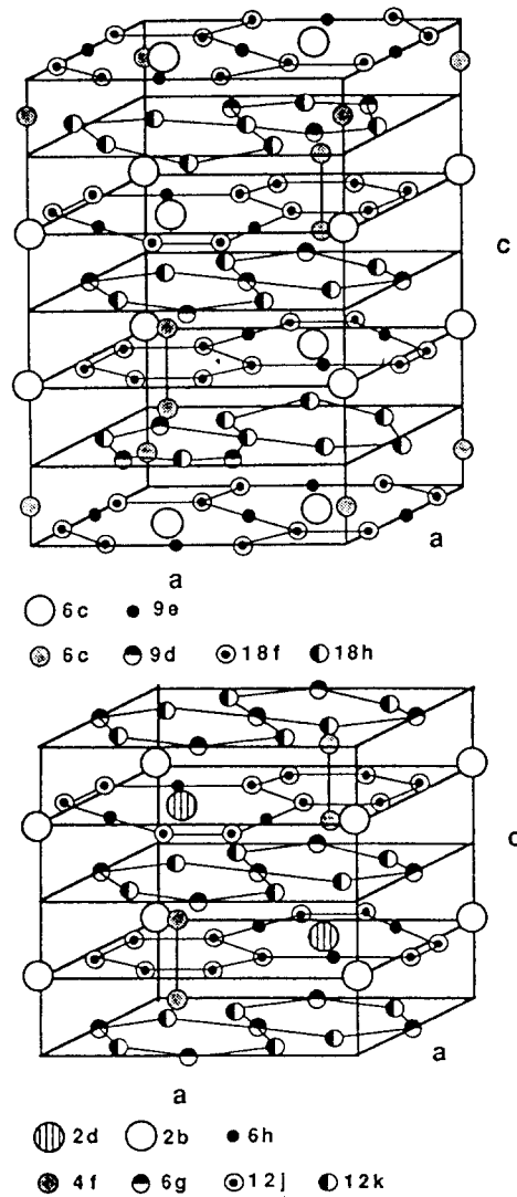
그림 1. Th_2Zn_{17} 왼쪽과 Th_2Ni_{17} (오른쪽)의 구조 Fig. 1. Th_2Zn_{17} (upper) and Th_2Ni_{17} (lower) structures
