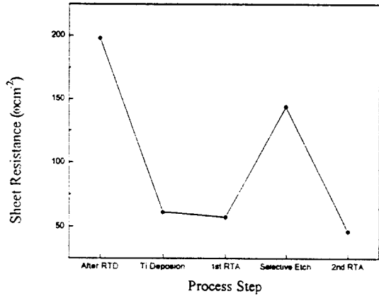
그림 2. RTD 공정 조건에 따른 면 저항
