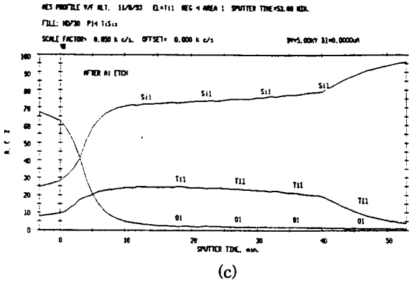
그림 3. 2차 RTA 온도 변화에 따른 AES 프로파일(RTD 공정조건 : 1050°C, 10초) (a)700°C, 30초 (b)750°C, 30초 (c)800°C, 30초
