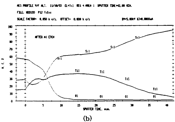
그림 4. 2차 RTA 시간 변화에 따른 AES 프로파일(RTD 공정조건 :1050°C, 10초) (a) 750°C, 10초 (b) 750°C, 60초
