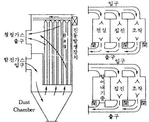
Fig. 7. 진동떨어내기방식 Bag Filter.
