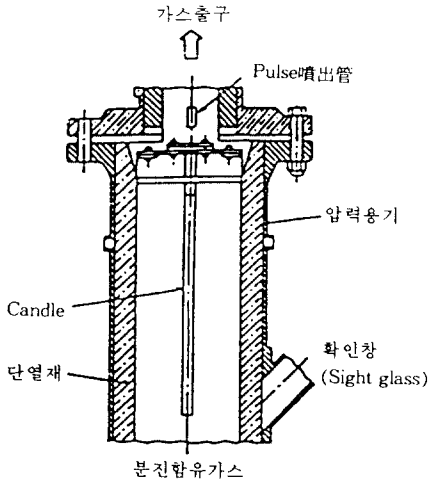
Fig. 2. Ceramic제 원통형 Filter(Candle Filter).
