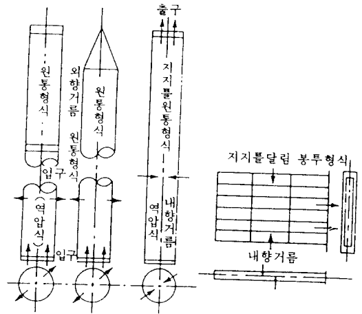
Fig. 4. Bag 형상과 여과방향.
