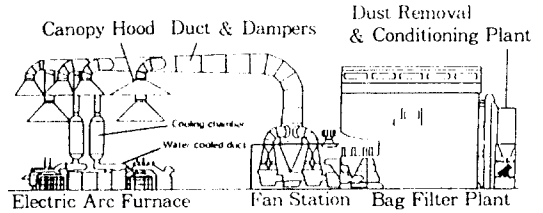
Fig. 15. 집진장치 계통도.
