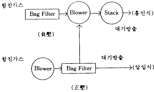
Fig. 5. 흡입식과 압입식의 Flow Sheet.
