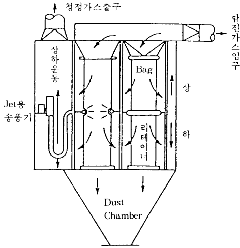
Fig. 10. Reverse Jet 탈어내기 방식의 Bag Filter.
