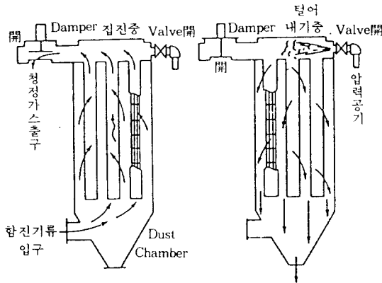
Fig. 11: 컴파아트먼트 Pulse 탈어내기 방식의 Bag Filter.
