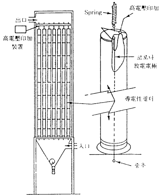
Fig. 17. 정전식 여과장치.
