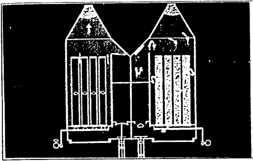
Fig. 18. 집진기 내부의 가스 흐름도.
