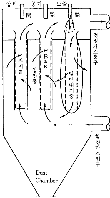
Fig. 9. Pulse Jet 털어내기 방식의 Bag Filter.
