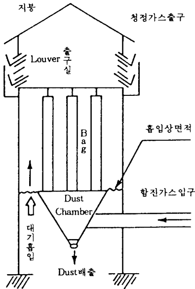
Fig. 6. 압입식 Bag Filter의 구조.
