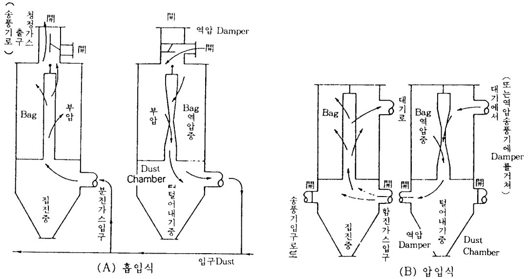
Fig. 8. 역압떨어내기 방식의 Bag Filter(흡입식과 압입식).
