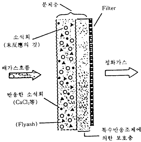
Fig. 14. 탈염·탈황·집진기구도.
