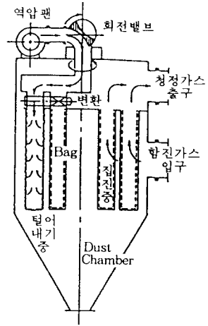
Fig. 12. 진동역압 탈어내기 방식의 Bag Filter.
