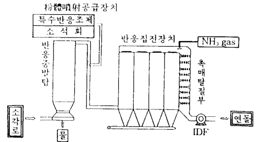
Fig. 13. Process의 Flow Sheet.
