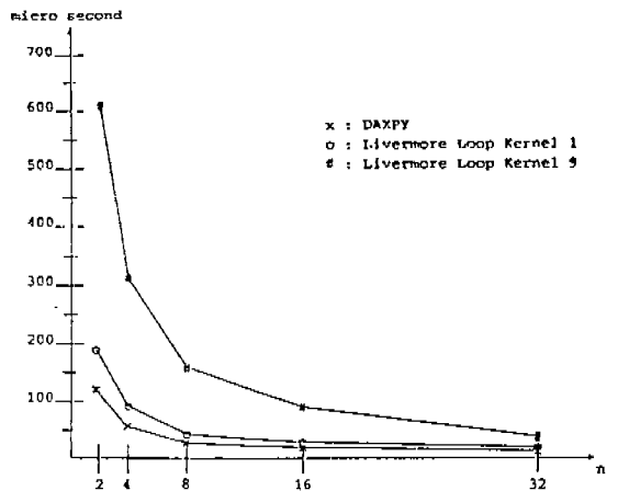
(그림 18) (그림17)의 수행시간 그래프 (fig. 18) Execution time graph of (Fig.17)
