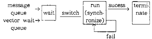
(그림 8) SP의 상태전이도 (Fig. 8) State transition diagram of SP
