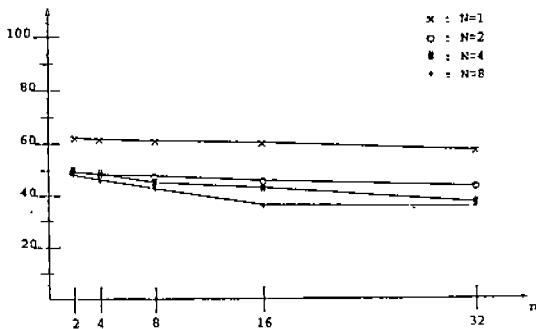
(그림 16) DP의 이용율 (Fig. 16) Utilization graph of DP
