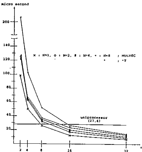
(그림 13) m=128 일때 수행시간 그래프 (Fig. 13) Graph of execution time for m=128
