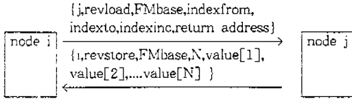
(그림 6) 벡터데이터의 revload,revstore 수행 (Fig. 6) Revload,revstore execution of vector data
