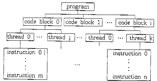
(그림 1) 프로그램 구조 (Fig. 1) Program structure
