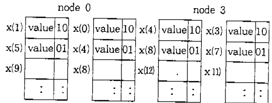
(그림 12) 저장후의 vector memory format (Fig. 12) Vector memory format after store
