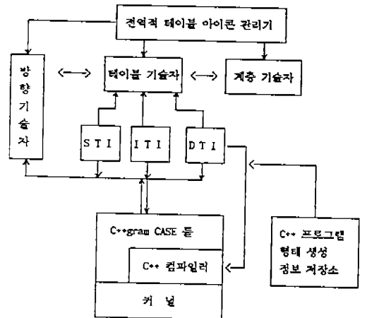
(그림 9) 시스템 구성도 (Fig. 9) System Configuration
