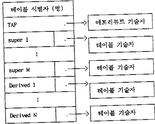
(그림 12) 계층 기술자 (Fig. 12) Hierarchy Descriptor
