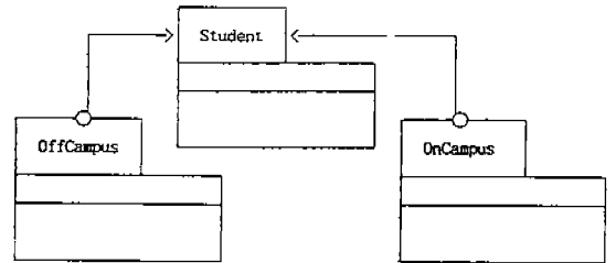
(그림 3) 클래스의 관계성 표기 예 (Fig. 3) Example of Class Relationship
