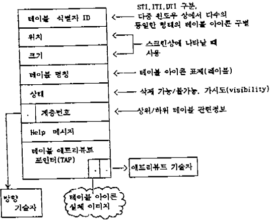
(그림 10) 테이블 기술자 (Fig. 10) Table Descriptor
