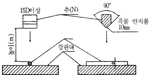
그림 내충격 시험장치
