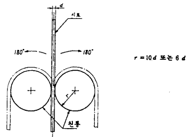
그림 굽힘 시험장치
