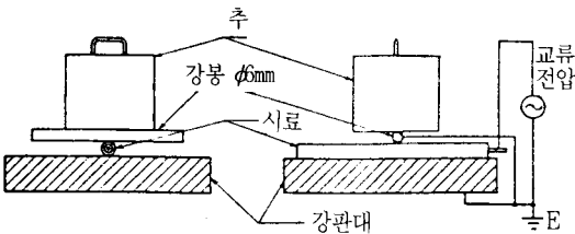
그림 내하중 시험장치
