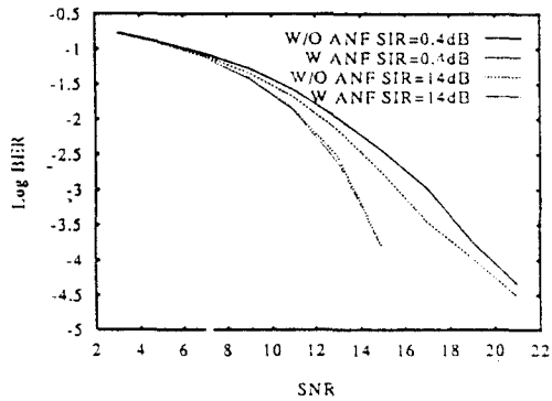
그림 16. PAM DFE에서 적응 노이즈캔서를 사용한 경우와 사용하지 않은 경우의 BER W/O ANF:ANF를 사용하지 않은 경우 W ANF:ANF를 사용한 경우
