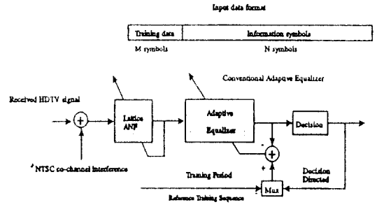
그림 7. 적응 도차판타를 사용한 NTSC 동원채널 간섭제거 시스템
