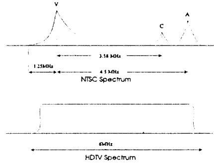
그림 6. NTSC 동원채널 간섭모형
