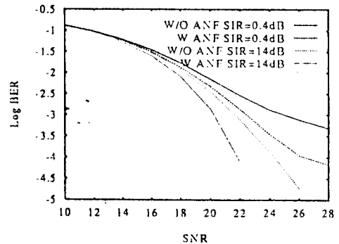
그림 14. QAM 변형등화기에서 ANF를 사용한 경우와 사용하지 않은 경우의 BER W/O ANF:ANF를 사용하지 않은 경우, W ANF:ANF를 사용한 경우
