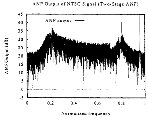
그림 13. 두단의 노치필터를 통과한 NTSC spectrum BER of QAM equalizer W or W/O ANF for NTSC interference
