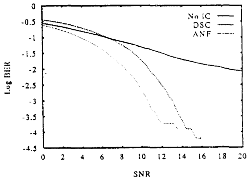
그림 17. 방송파의 주파수변이가 없을때 DSC-HDTV와 제안한 방식과의 BER 성능비교(C/I=20dB)
