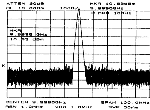
그림 10. 위상고정 유전체 공진 발진기의 주파수 응답 (Span=100 MHz)
