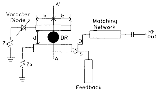
그림 4. 전압제어 유전체 공진 발진기의 구성 Fig. 4. Configuration of the VCDRO
