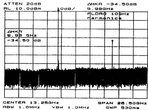
그림 14. 위상고정 유전체 공진 발진기의 고조파와 스퓨리어스 특성
