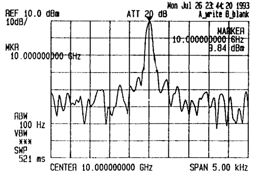
그림 13. 위상고정 유전체 공진 발진기의 주파수 응답 Span 5 KHz (ADVANTEST MS2702A)
