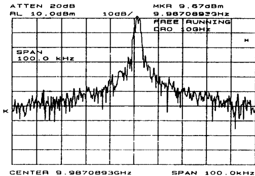
그림 11. 전압제어 유전체 공진 발진기의 주파수 응답 (Span=100 KHz)
