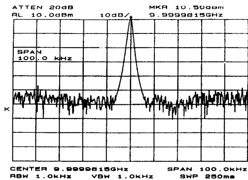
그림 12. 위상고정 유전체 공진 발진기의 주파수 응답 (Span=100 KHz)
