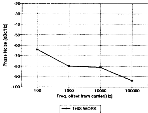
그림 15. 위상고정 유전체 공진 발진기의 위상 잡음 특성
