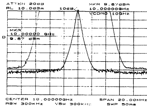
그림 7. 진압제어 유전체 공진발진기의 튠링된 스펙트럼 Fig. 7. Tuned spectrum of the VCDRO
